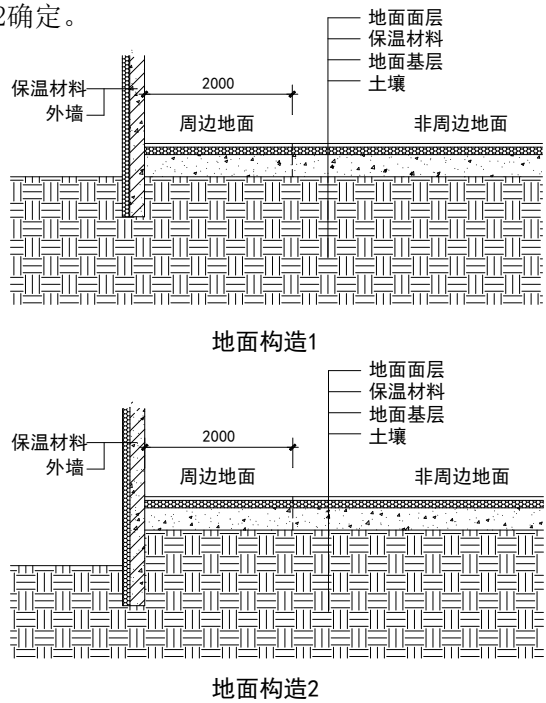
图 C. 0. 3 典型地面构造示意图
