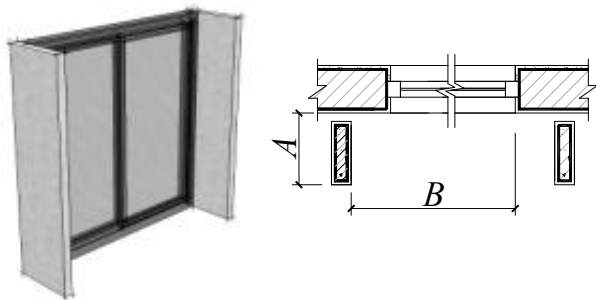
图 D.0.1-2 垂直遮阳的特征值的示意
