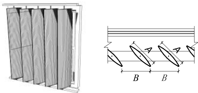
图 D.0.1-5 竖百叶挡板式遮阳的特征值的示意
