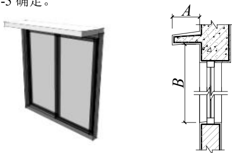
图 D.0.1-1 水平遮阳的特征值的示意
