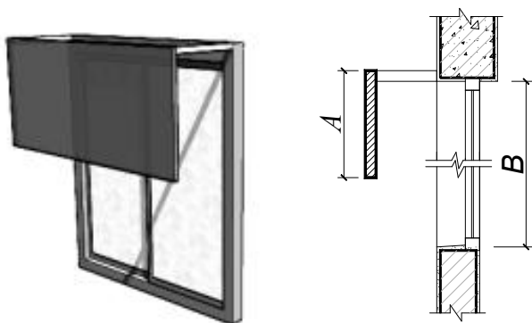
图 D.0.1-3 挡板遮阳的特征值的示意
