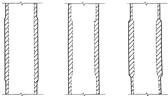
图 5.2.9-1 节点区柱管壁加厚示意图
