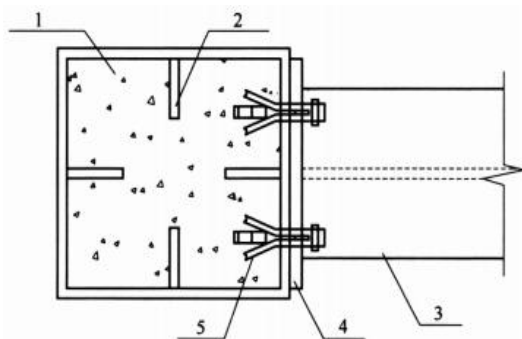
图 5.2.9-2 柱管壁内部设置加劲肋示意图
