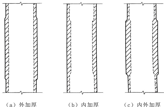
图 5.2.9-1 节点区柱管壁加厚示意图
