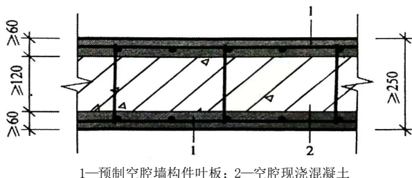
图 4.3.2 地下工程叠合外墙平面示意图
