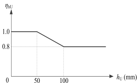
图 3.1.6 构件厚度影响系数
