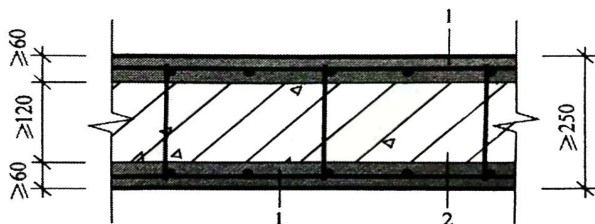
图 4.3.2 地下工程叠合外墙平面示意图
